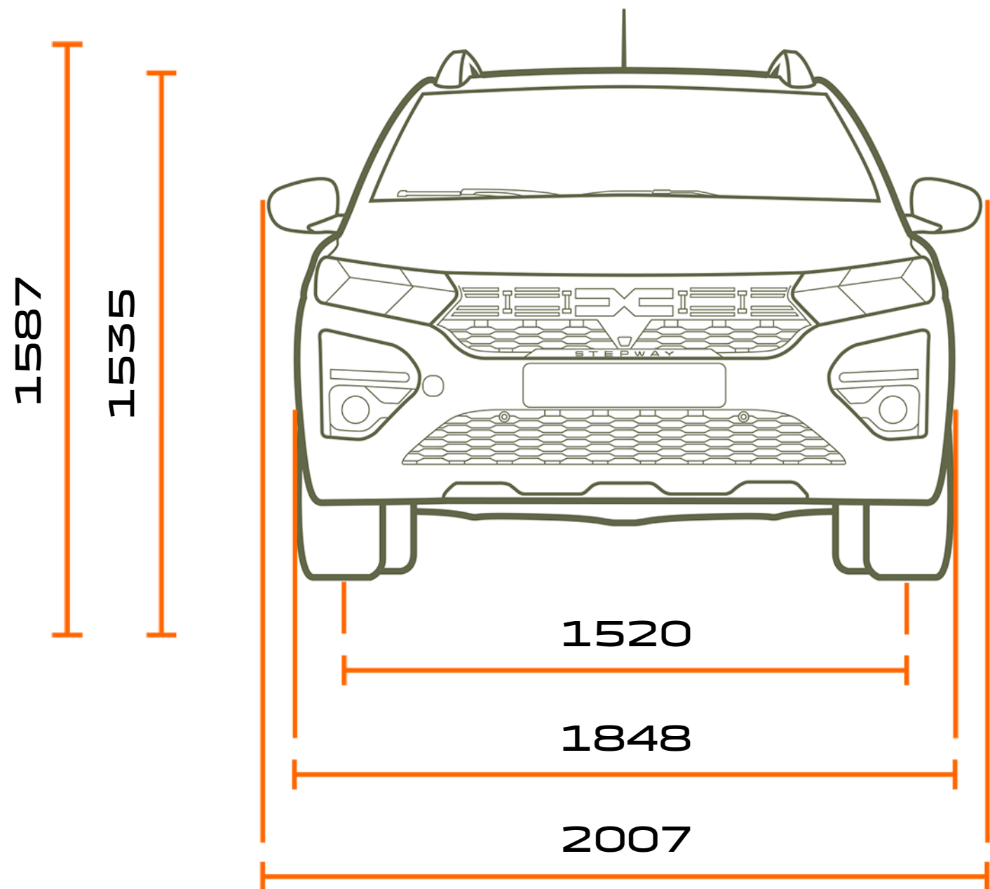
VAADE EEST
