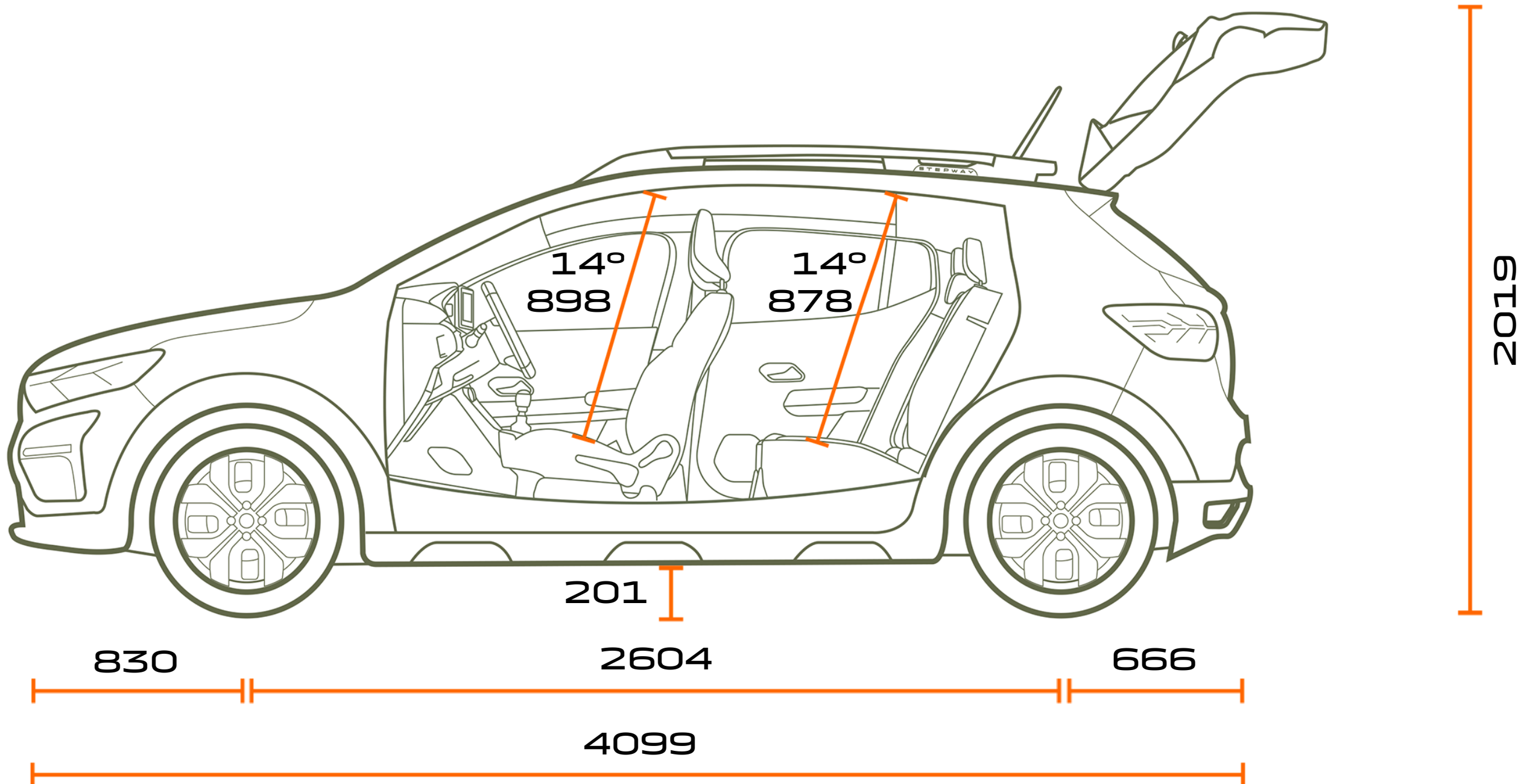
VAADE KÜLJELT
